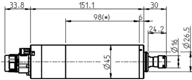
寸法図
