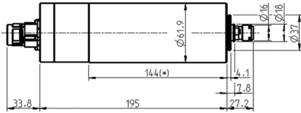
寸法図
