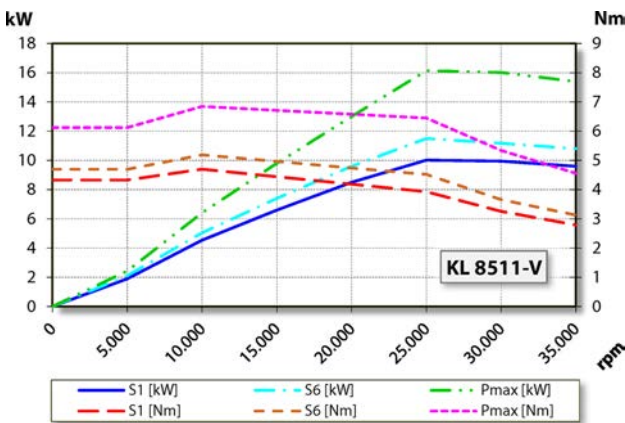
Diagramma di potenza Raffreddato a liquid
