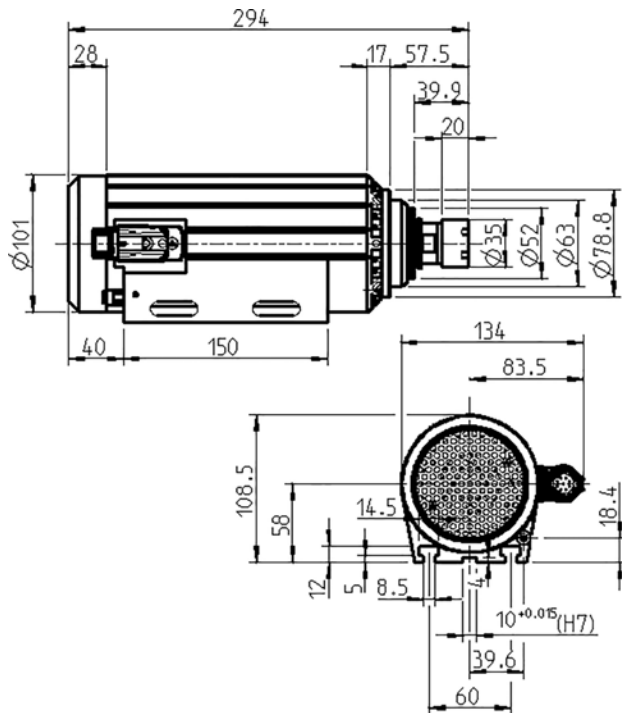
寸法図
