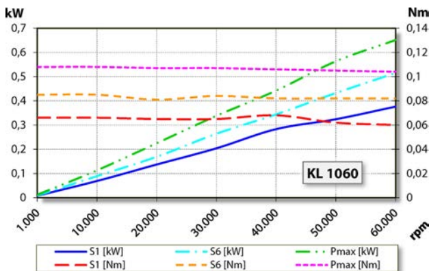
Vermogensdiagram
