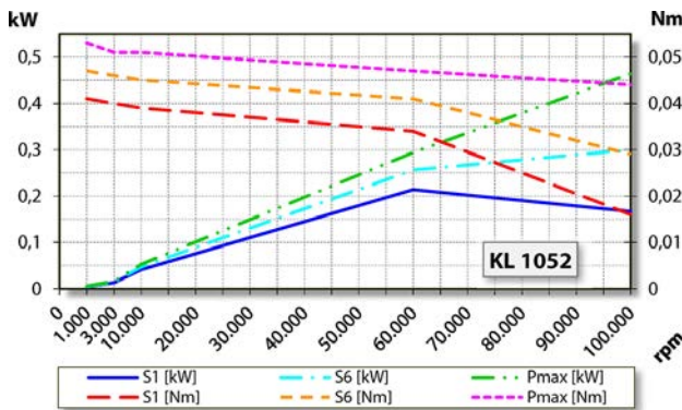
出力、トルク-回転数ダイヤグラム 圧縮空気冷却
