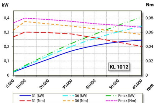
Diagram výkonu Nechlazen
