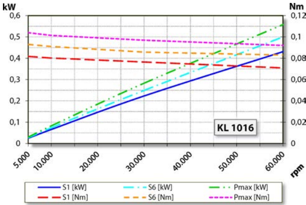
Güç diyagramı Mil tutucusu soğutulmuş
